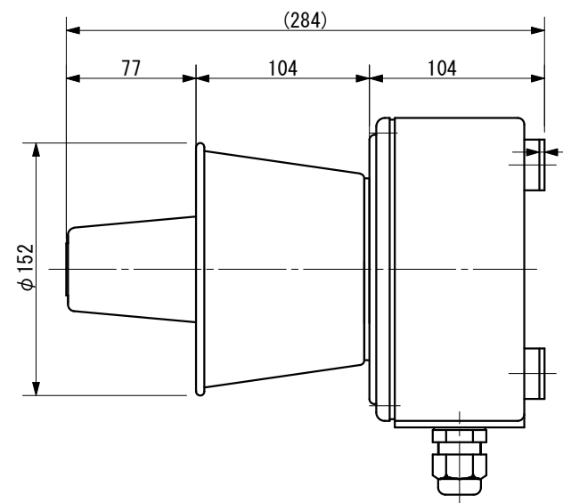
CABLE GLAND / ケーブルグランド
